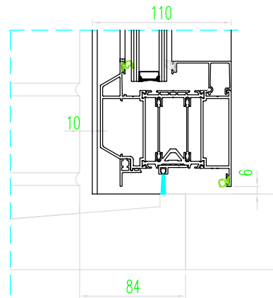
Dorpelaansluiting deur met borstel
