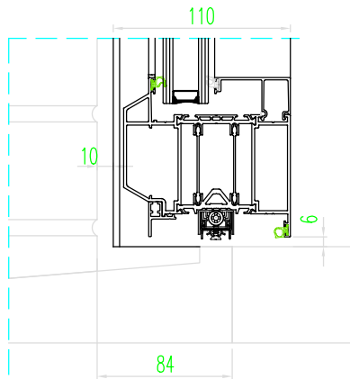
Dorpelaansluiting deur met dalende drempel
