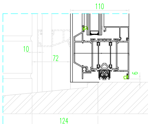
Dorpelaansluiting deur met rolluikgeleider met dalende drempel
