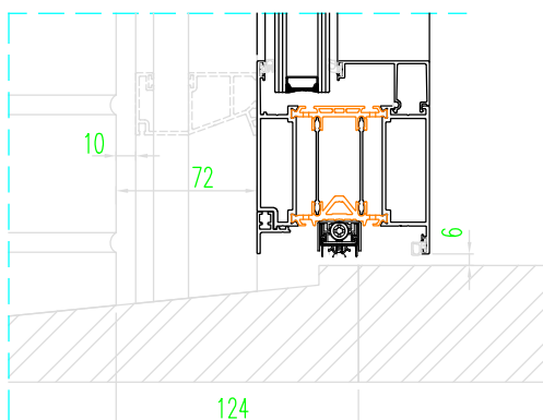
Dorpelaansluiting deur met rolluikgeleider met dalende drempel
