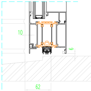
Dorpelaansluiting deur met dalende drempel
