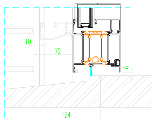
Dorpelaansluiting deur met borstel met dalende drempel
