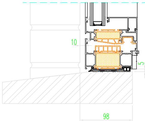
Dorpelaansluiting op rubber Systeem A
