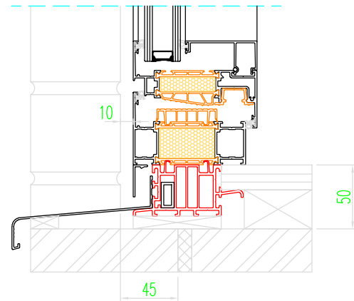
Dorpelaansluiting met alu dorpel Systeem C
