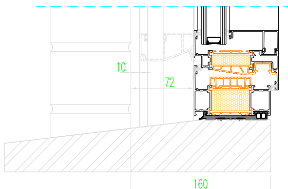
Dorpelaansluiting met rolluikgeleider
