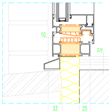
Dorpelaansluiting met renovatieneusje Systeem E
