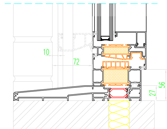
Dorpelaansluiting met rolluikgeleider Systeem G
