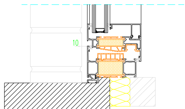
Dorpelaansluiting Systeem F
